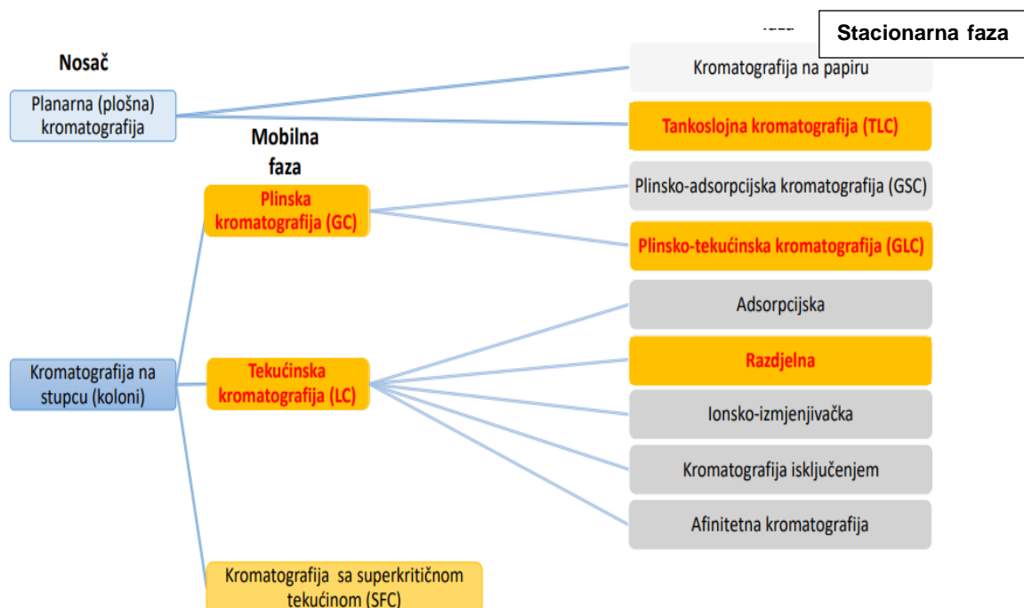
Slika 3.1: Podjela kromatografije
