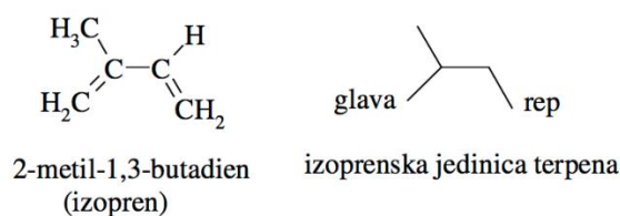
Slika 2.1. Strukturna formula izoprena i prikaz izoprenske jedinice
