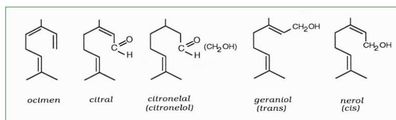
Slika 2.2. Aciklički monoterpeni
