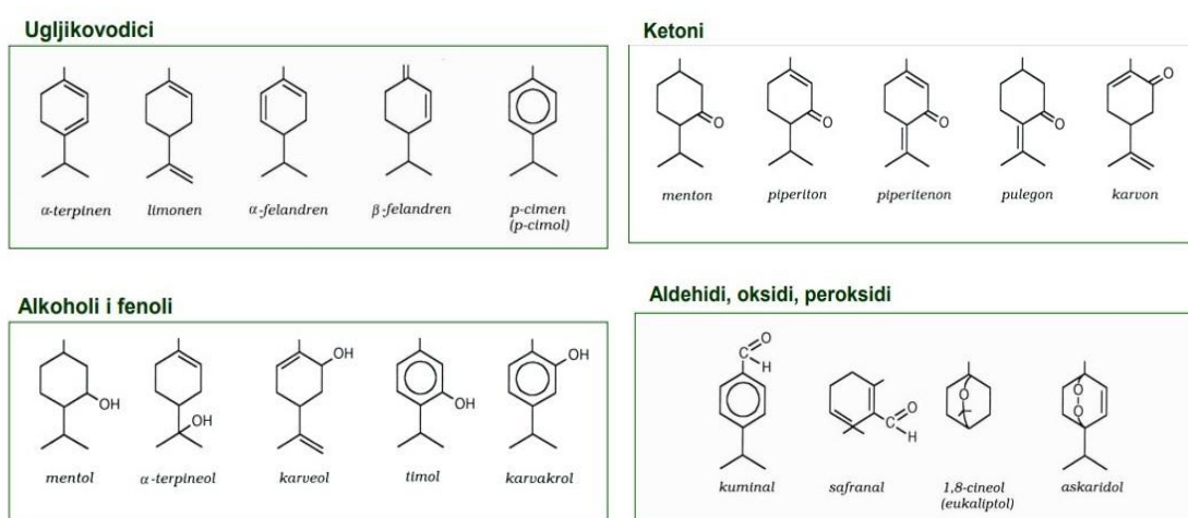
Slika 2.3. Monociklički monoterpeni
