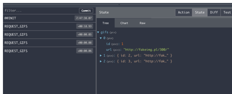
Slika 15. Redux DevTools 42
