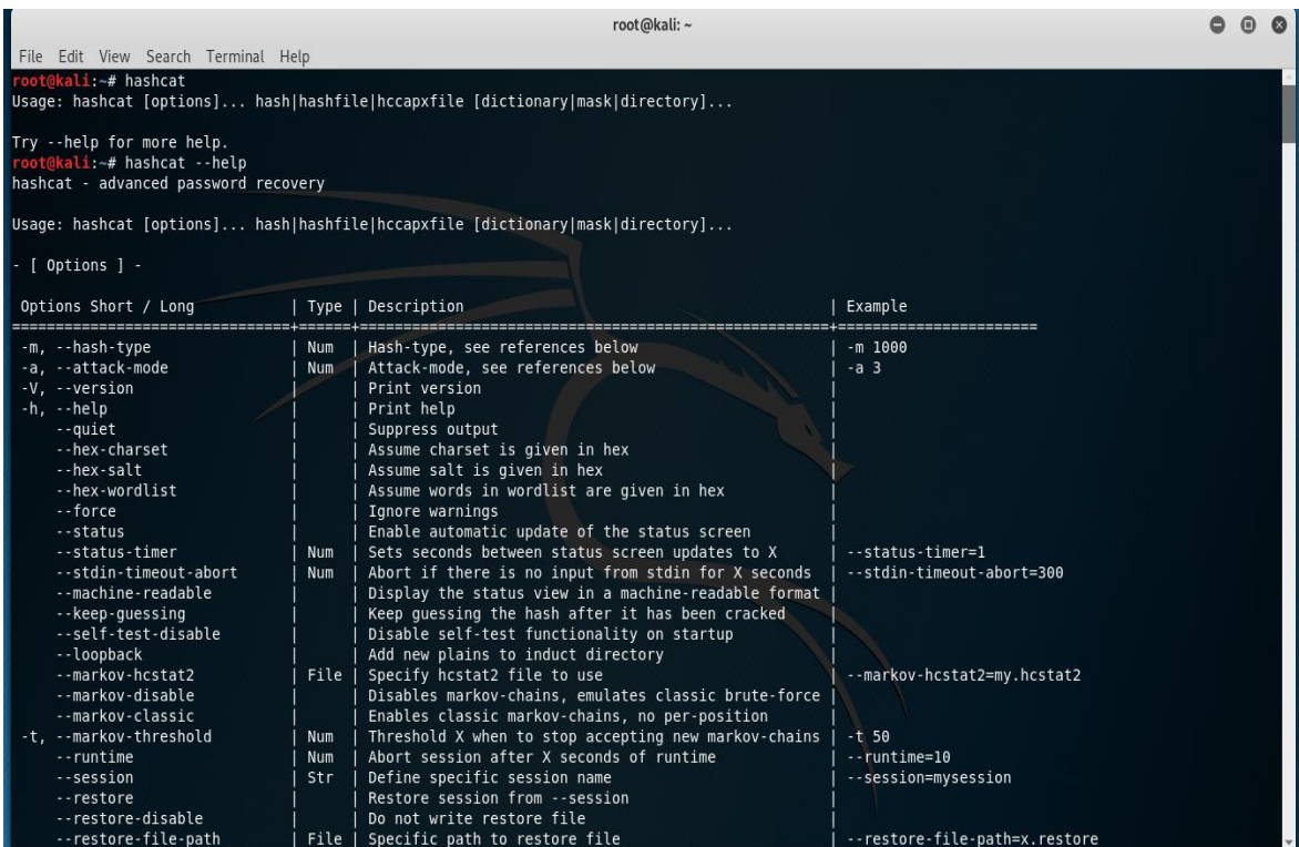
Slika 6-29 Hashcat alat za probijanje zaporki
