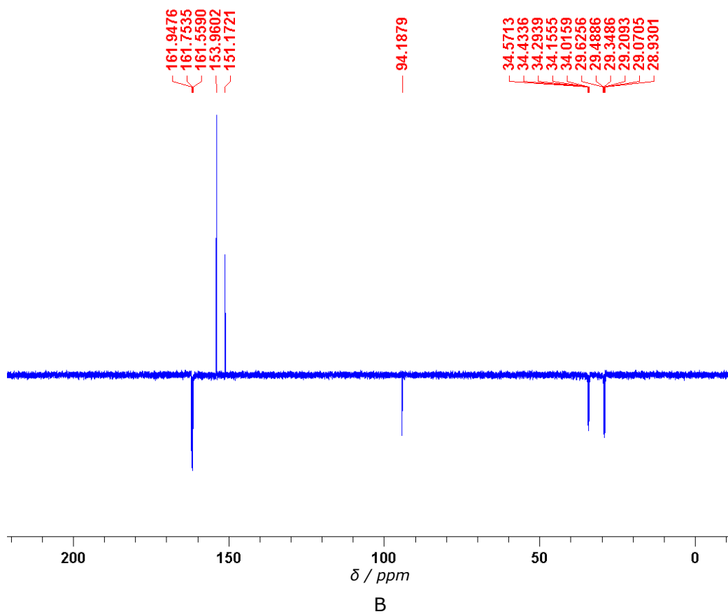
Slika D9. A) 1 H spektar i B) 13 C spektar L2.
