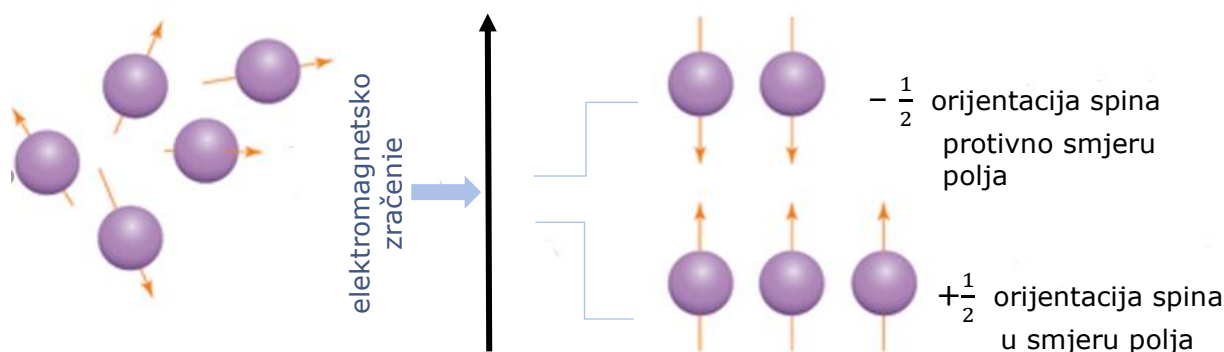
Slika 13. Orijetacija spina nakon djelovanja vanjskog magnetskog polja.
