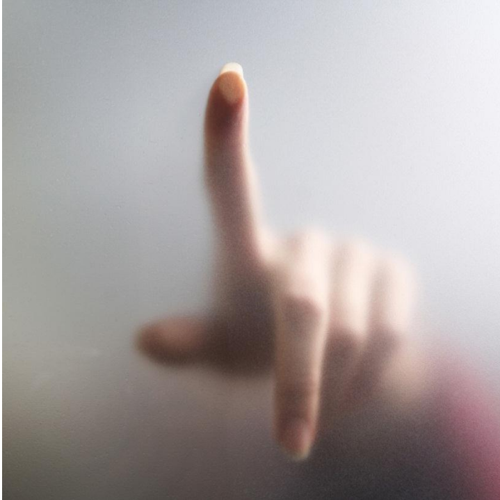
Slika 6: Osjetilo dodira
