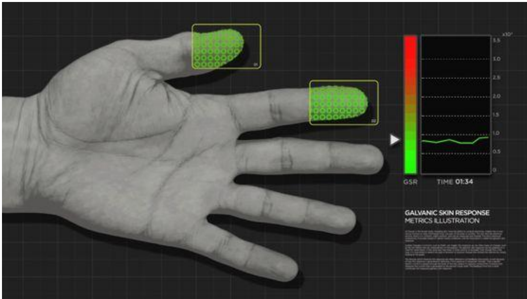
Slika 8: GSR
