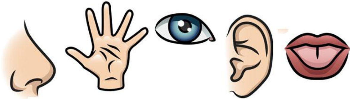
Slika 1: 5 osjetila
