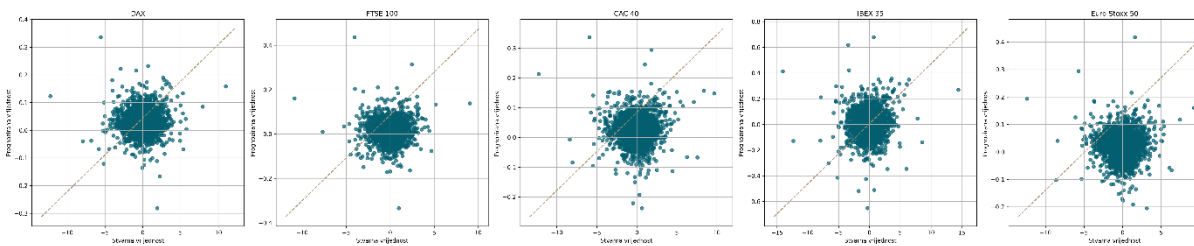
Slika 24 Dijagram raspršenosti za AR(4) model
