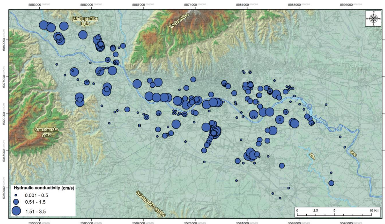
Slika 9. - Hidraulička vodljivost šireg zagrebačkog područja
