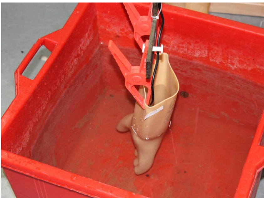
Sl. 3.15. Dielektrično ispitivanje izolacijske rukavice za RPN
