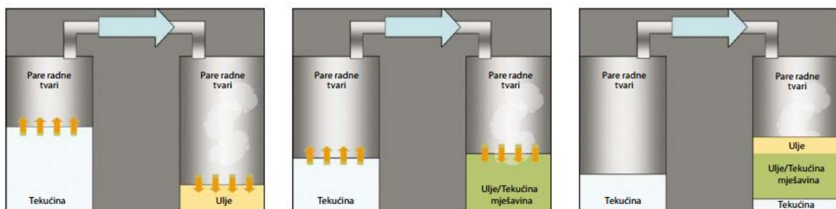
Slika 13: Kondenziranje radne tvari unutar kompresora [25]
