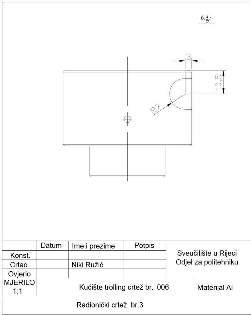
Slika 4.10. Prikaz tehničkog crteža (3)
