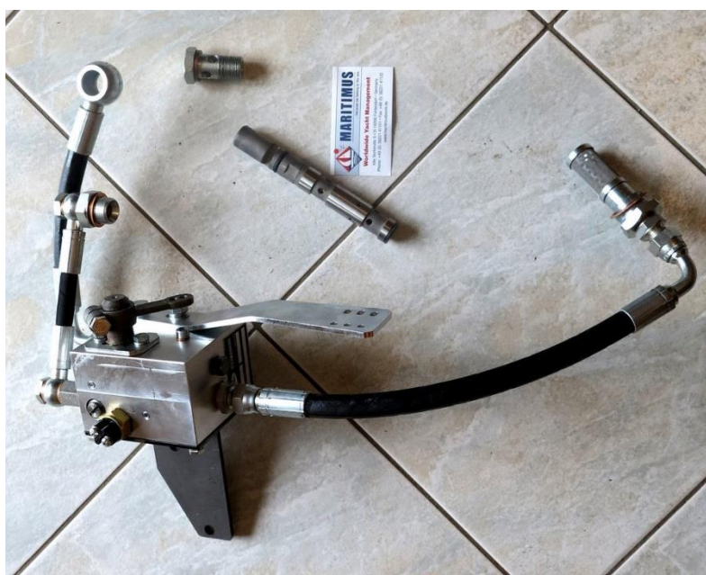
Slika 2.3. Trolling ventil tvrtke „Maritimus“
