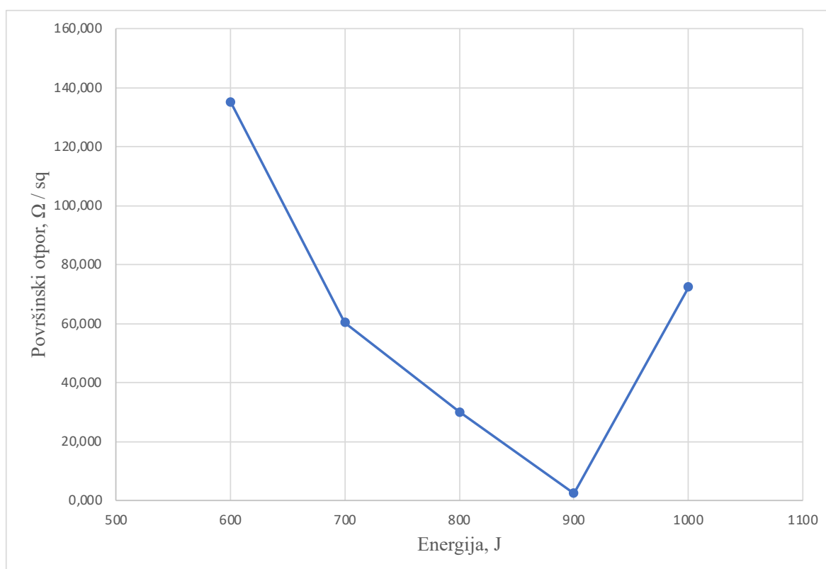
Slika 4.37. Grafički prikaz rezultata preliminarnih ispitivanja amfifilne tinte na ABS podlozi.
