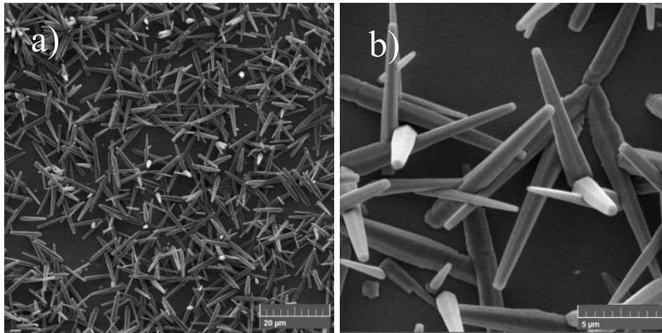
Slika 21. SEM mikrografije nanoštapića s bazom vode dobivenih hidrotermalnom metodom
