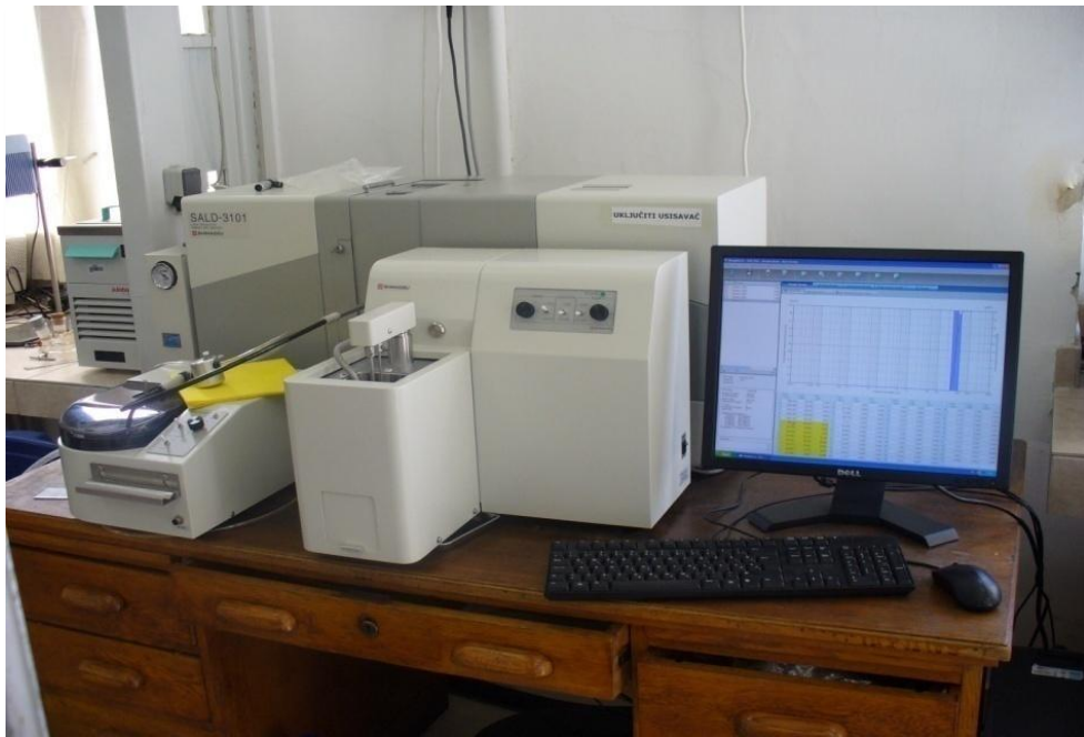
Slika 3.3. Fotografija uređaja za određivanje raspodjele veličine čestica metodom laserske difrakcije SALD – 3101 (Shimadzu, Kyoto, Japan).
