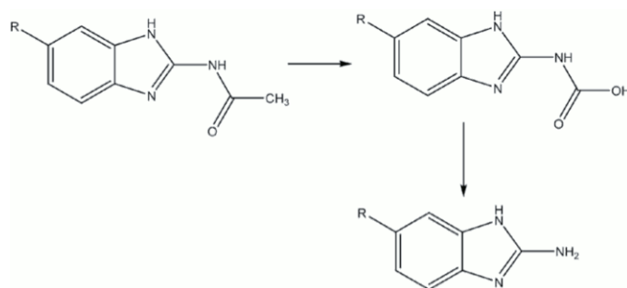
Slika 1. Fotorazgradnja benzimidazolnih antihelminatika [12]
