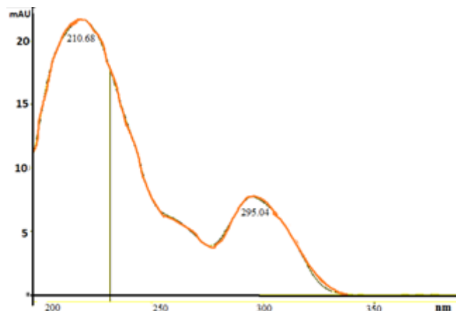
Slika 24. Apsorpcijski spektar albendazola na 210 nm u standardnoj otopini 10 mg/L
