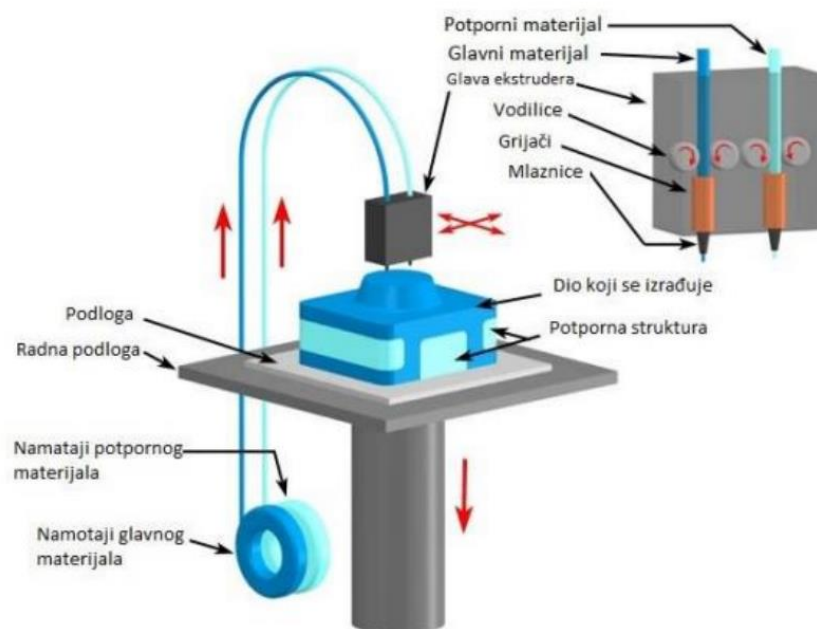
Slika 8. Izrada modela postupkom taložnog sraščivanja [22]
