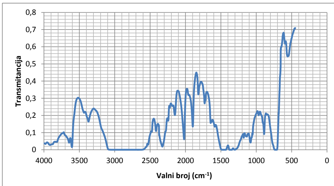
Slika 64. Spektar PE folije debljine 1000 µm, transmisijnska metoda.
