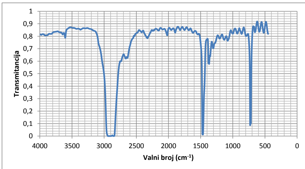
Slika 62. Spektar PE folije debljine 50 µm, transmisijaska.
