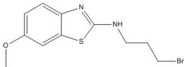
Slika 10. Struktura (3-bromopropil)-(6-metoksibenzotiazol-2-il)amina
