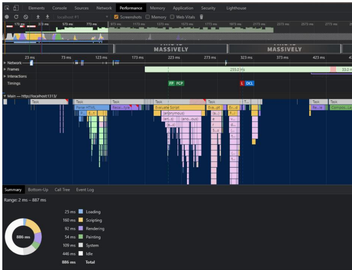
Slika 16. Rezultati testa performansi brzine Hugo okvira
