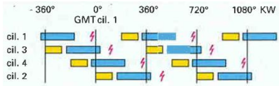
Slika 15. Slijedno ubrizgavanje
