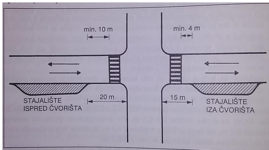
Slika 6. Stajališta za zaustavljanje autobusa
