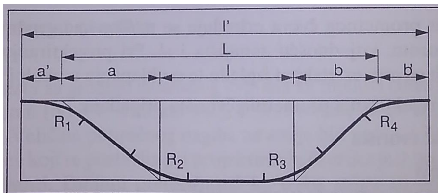
Slika 7. Polumjeri zaobljenja prilaza autobusnom stajalištu
