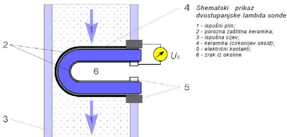
Slika 4.4 Prikaz rada lambda sonde [10]
