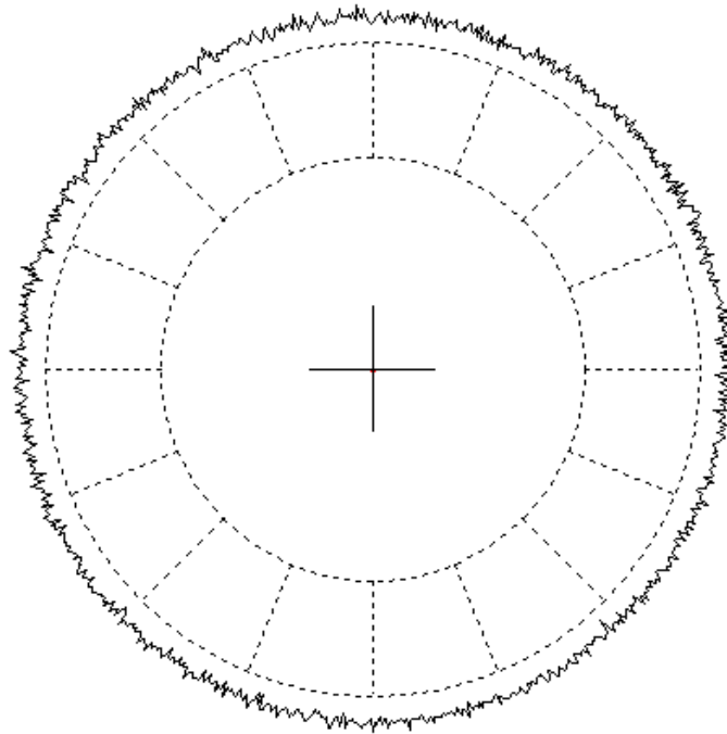
Slika 51. Prikaz nasumično odabranih brojeva normalnom razdiobom za mjesto područje \pm 10 \mu\text{m}
