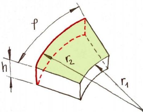
Slika 59. Geometrija kandže
