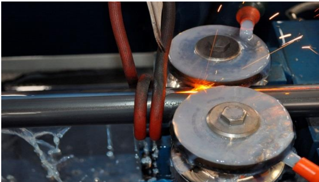
Slika 10. Indukcijsko zavarivanje [11]
