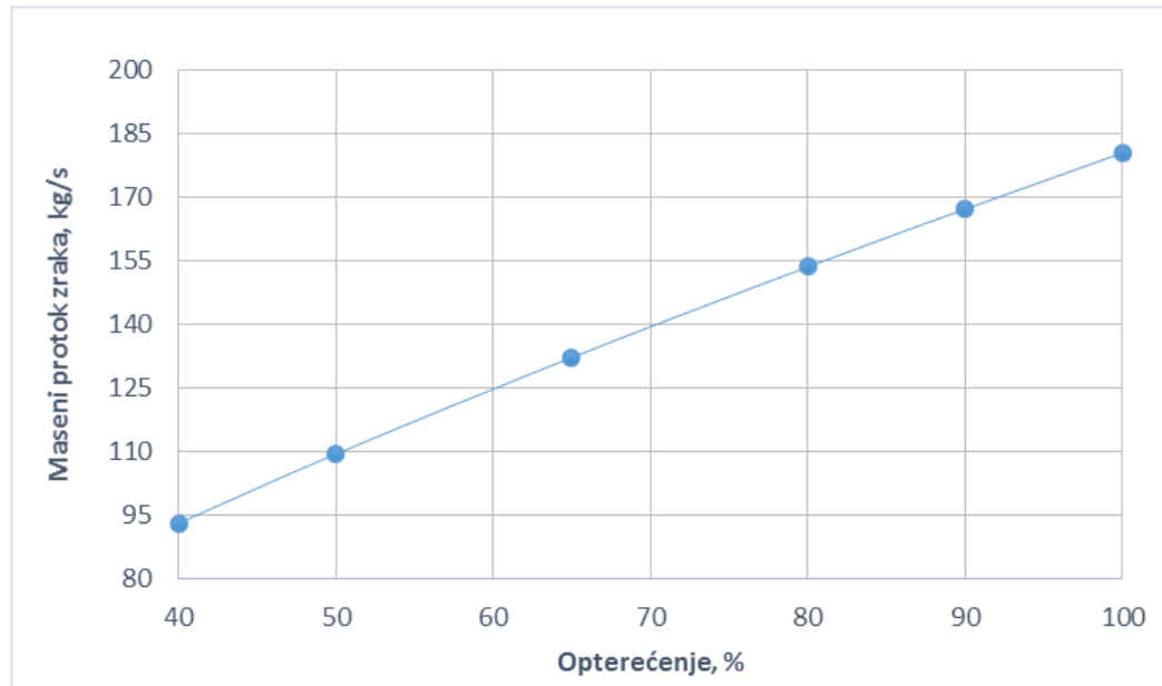
Slika 37. Promjena masenog protoka zraka modela s izmjenjivačem otpadne topline s promjenom opterećenja
