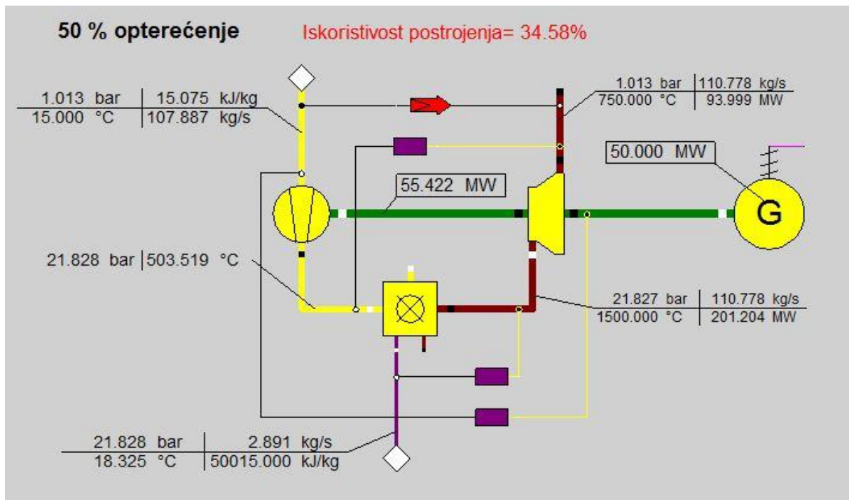
Slika 23. Osnovni model plinskoturbinskog postrojenja u EBSILON -u pri opterećenju od 50 %
