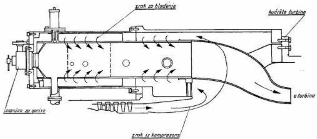
Slika 5. Komora izgaranja [1]
