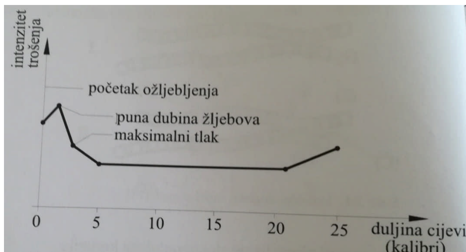
Slika 5.1. Dijagram trošenja cijevi [1]
