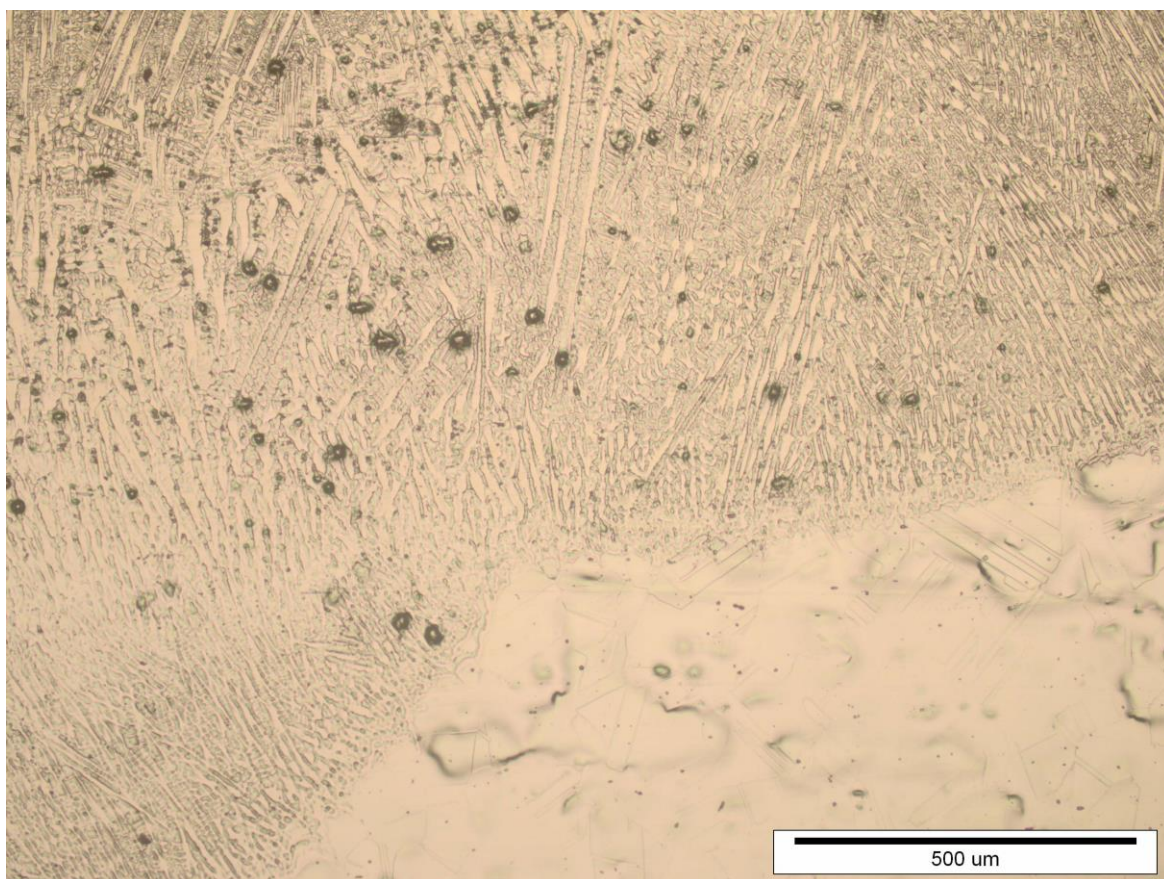
Slika 16. Prikaz zarobljenih uključaka u metalu zavara [26]
