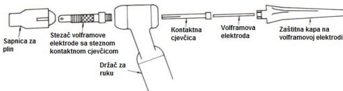
Slika 9. Shematski prikaz zrakovog hladnog pištolja [21]
