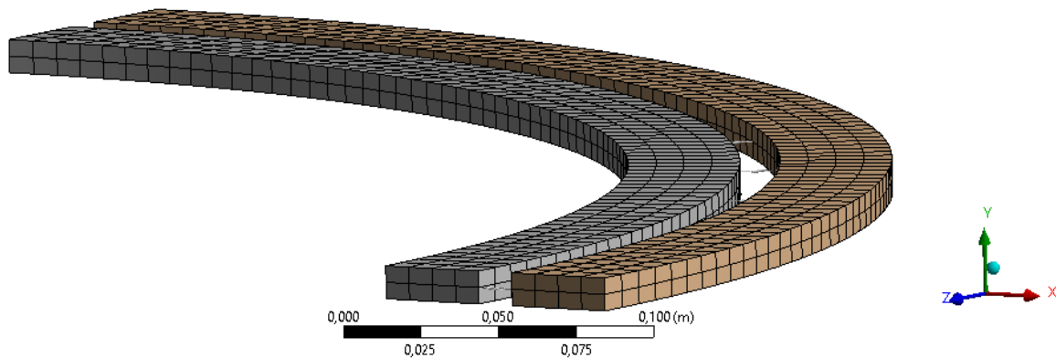
Slika 36. Mreža konačnih elemenata detaljnog modela jednog sloja vodiča NN namota (1 272 elementa)
