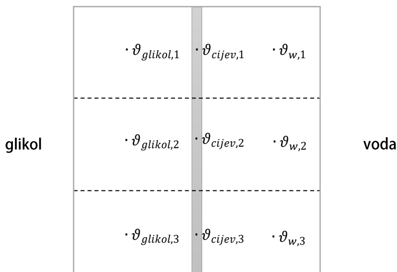
Slika 8. Diskretizirani model toplinskog spremnika
