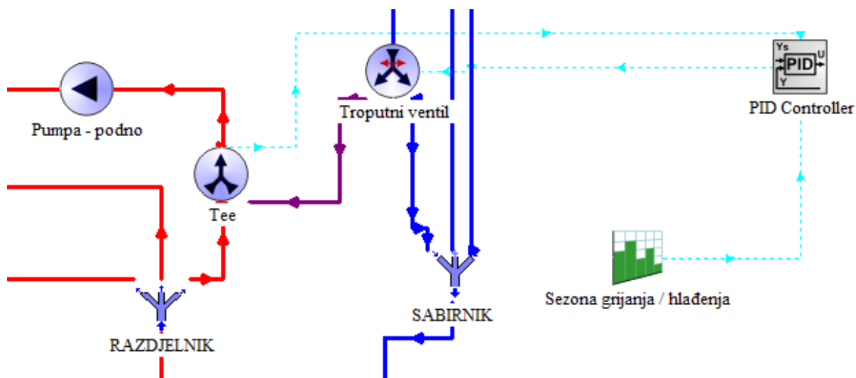
Slika 44. Model regulacije troputnog ventila
