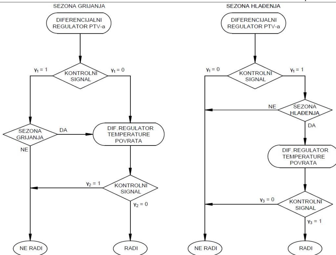
Slika 38. Dijagram toka regulacije dizalice topline u režimu grijanja (lijevo) i hlađenja (desno)
