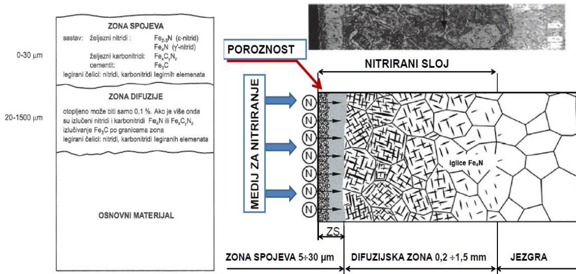
Sl. 29 Prikaz nitriranih slojeva [16]
