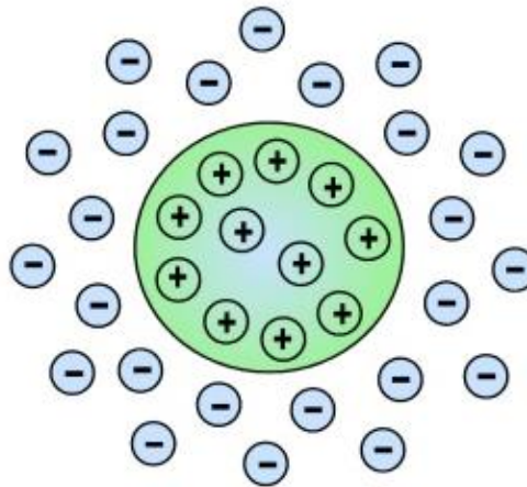
Slika 16. Elektrostatička stabilizacija [25]
