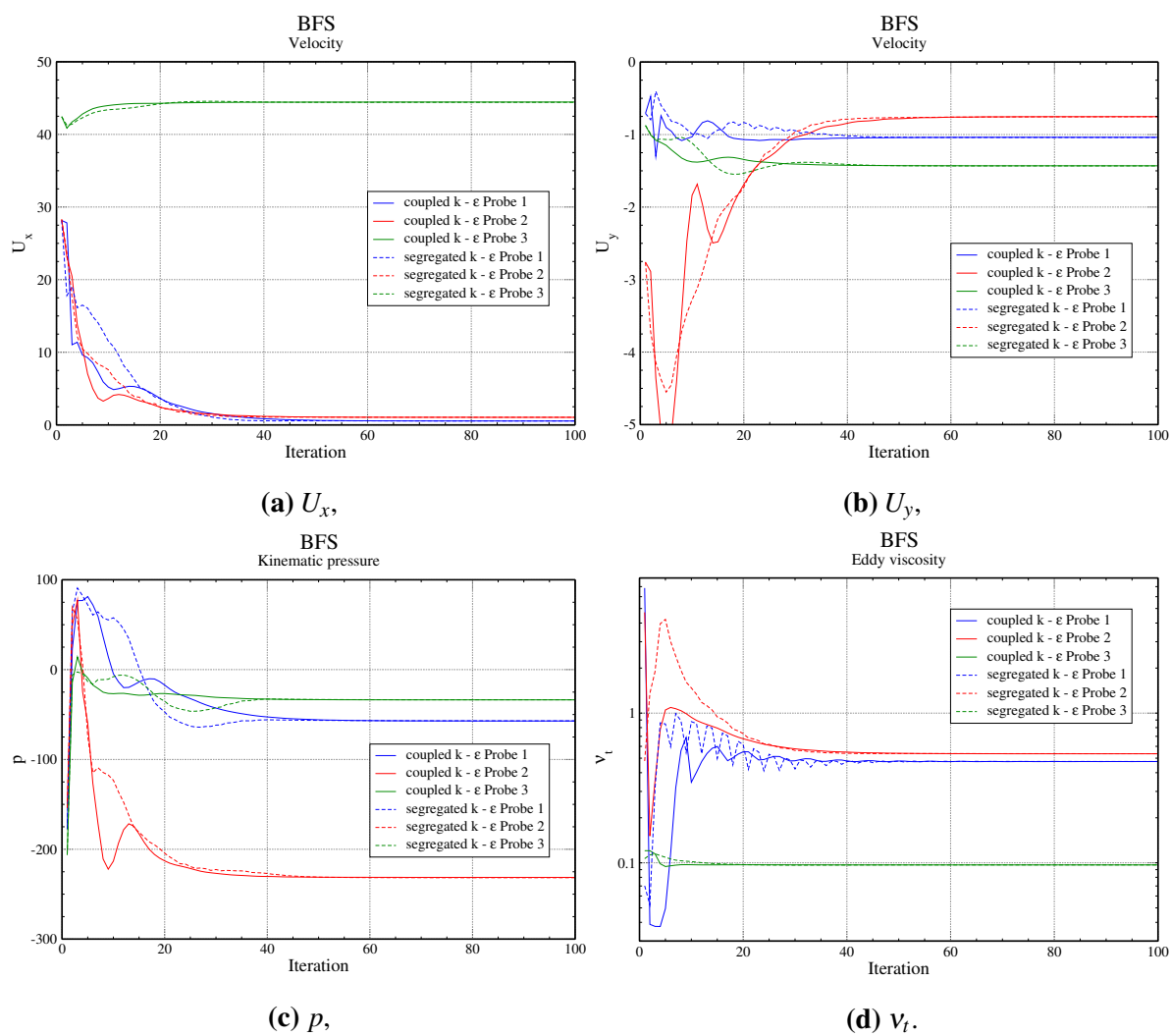
Slika 10: BFS: Usporedba konvergencije vrijednosti polja implicitno spregnutog i odvojenog k - \varepsilon modela turbulencije.
