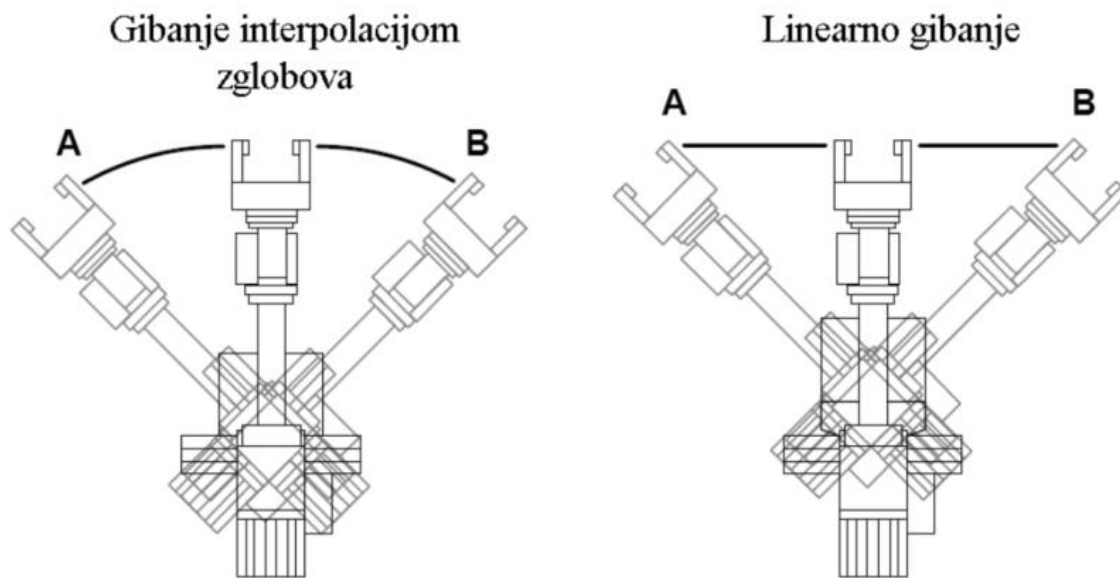
Slika 19. Vrste gibanja središta alata robota
