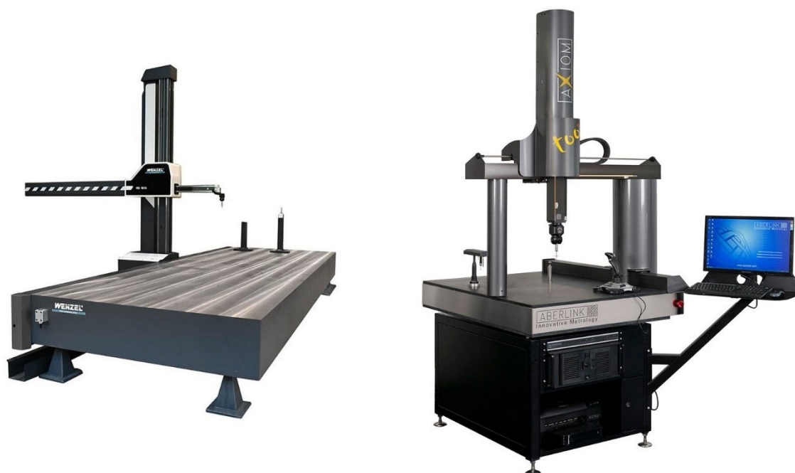
Slika 33. Koordinatni mjerni uređaj: horizontalni (lijevo) i vertikalni (desno) [23],[24]
