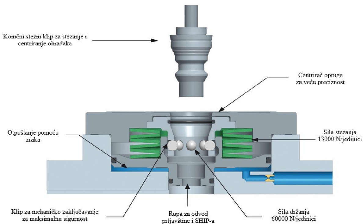
Slika 10. Stezni mehanizam [12]
