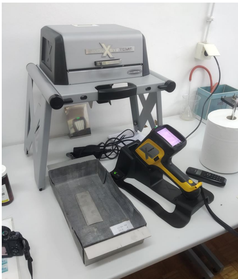
Slika 21. Oprema za analizu kemijskog sastava čelika
