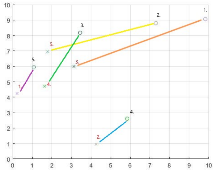
Slika 10. Rezultat FCFS algoritma
