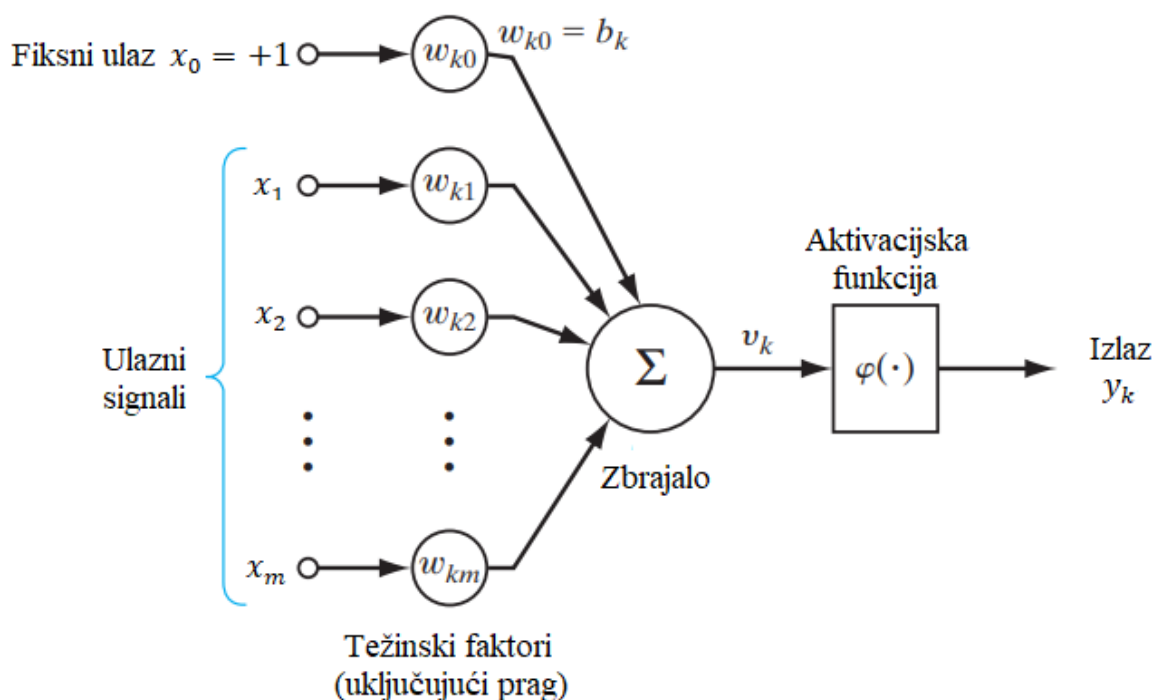
Slika 4 Nelinearni model neurona k s uračunatim pragom [14]
