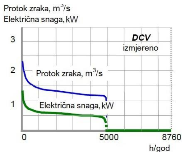
Dijagram 2: Sustav ventilacije s protokom zraka na zahtjev [1]
