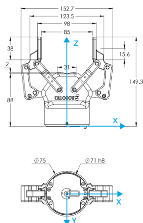
Slika 3.11 Dimenzije hvataljke Robotiq 2F-85 [28]
