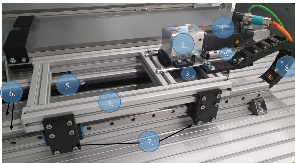
Slika 19. Finalna verzija konstrukcije. 1. – motor, 2. – reductor, 3. – 3D printani držač reduktora, 4. – aluminijska platforma, 5. – zupčasta letva, 6. – nosiva konstrukcija, 7. – vagoni na vodicama, 8. – IGUS energy chain, 9. – bumper
