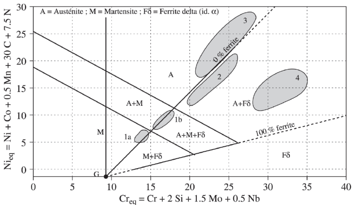
Slika 11. Zingg-Geiger-ov strukturalni dijagram lijevanih nehrđajućih čelika [16]
