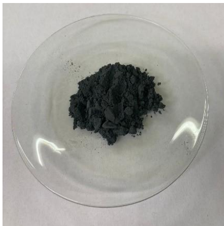
Slika 19. Nanočestice aluminija
