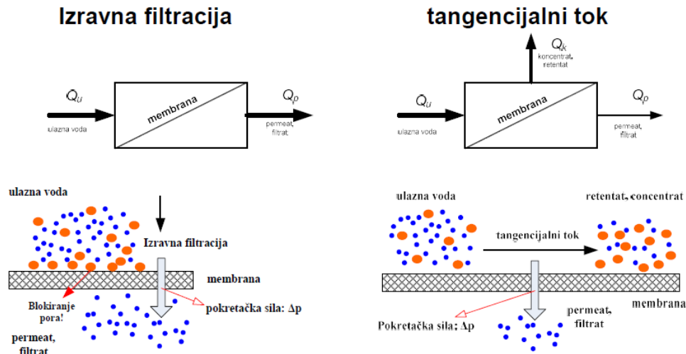
Slika 4. Načini rada membrane
