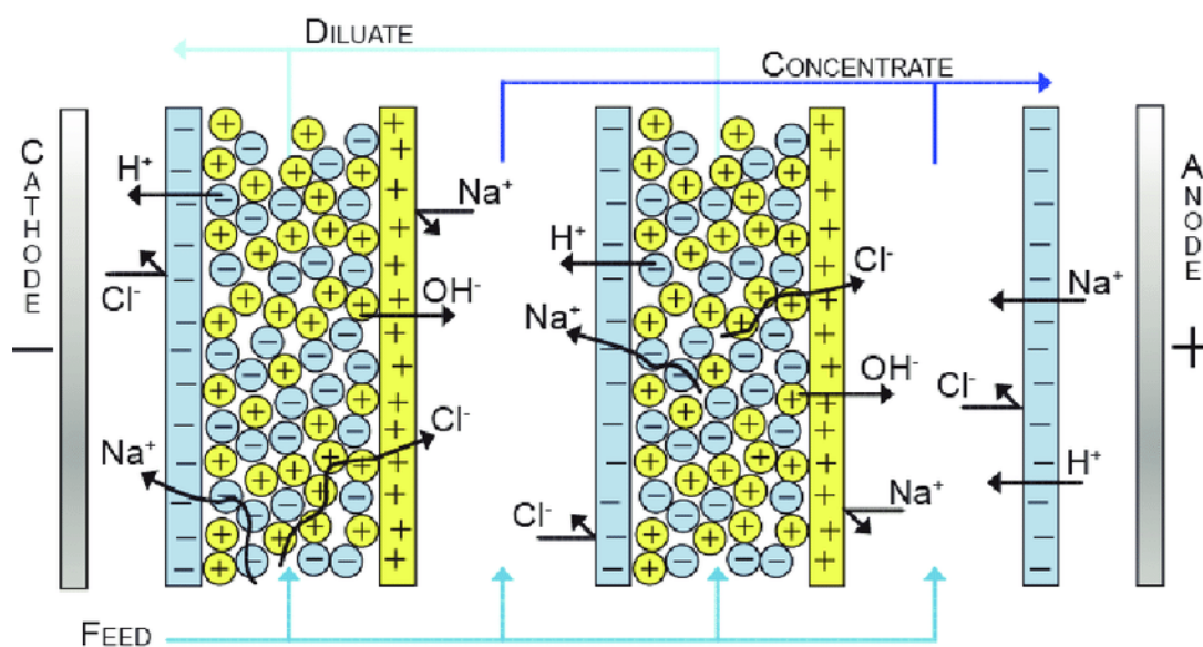
Slika 12. Shematski prikaz postupka elektrodeionizacije
