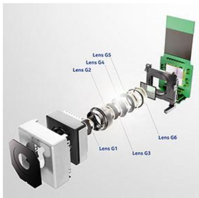
Slika 8. Fotoapararat mobitela [10]
