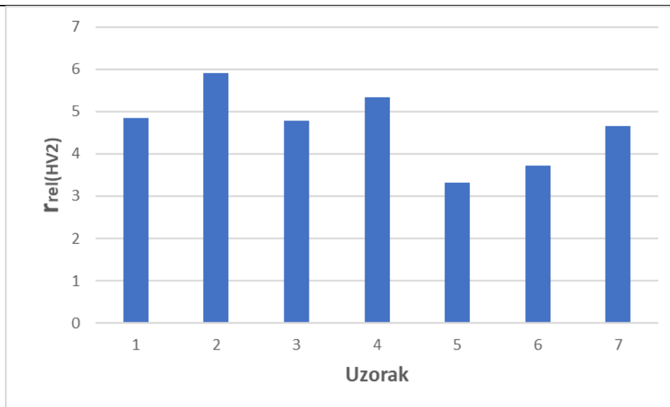
Slika 24. Dijagram nejednolikosti površinske tvrdoće za metodu HV2
