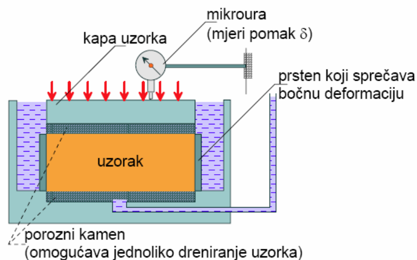
Slika 7. Shema edometra [6]
