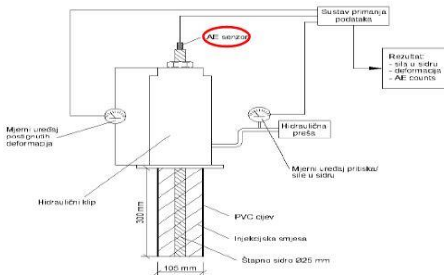
Slika 9. Akustična emisija [10]
