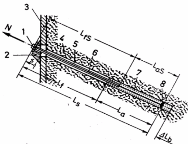
Slika 3. Elementi sidra [4]
